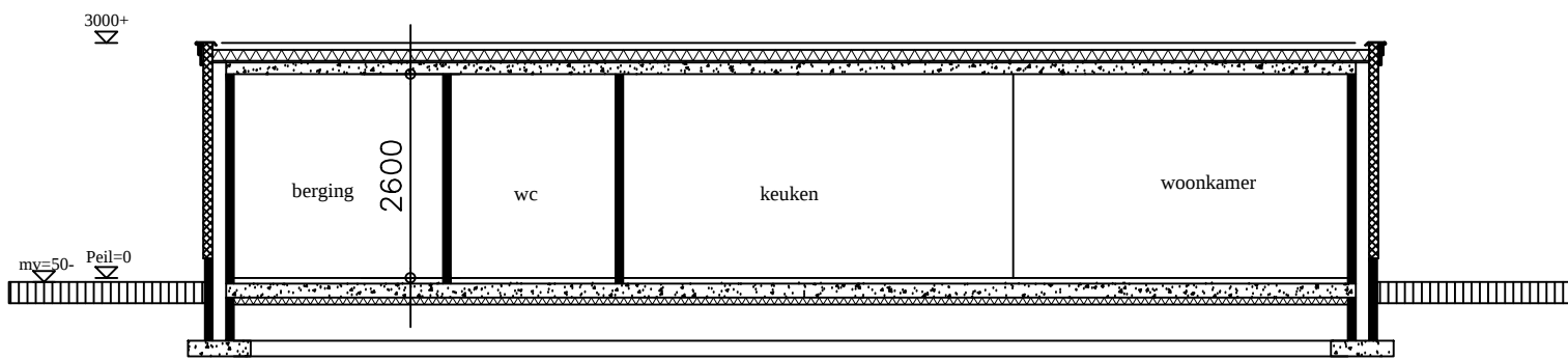
doorsnede A
