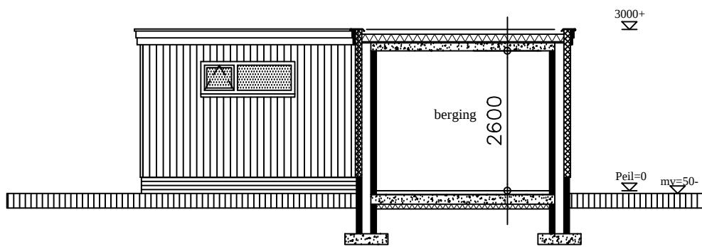
doorsnede C
