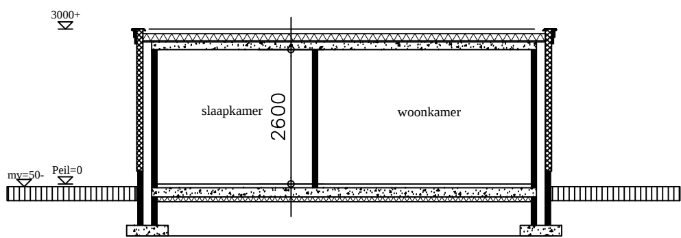
doorsnede D
